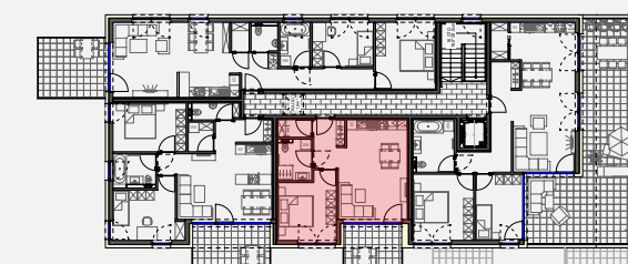
GRUNDRISS EBENE 3 / HAUS B M 1/500
